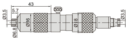
微分头(100-115mm)
